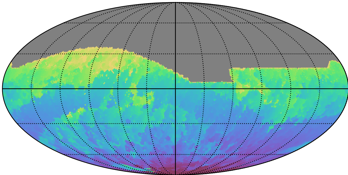
extra_ss_neo3_v3.4_10yrs All sky i band: Min HA
