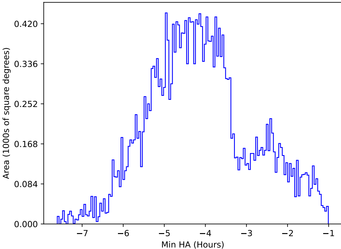
extra_ss_neo3_v3.4_10yrs All sky i band: Min HA
