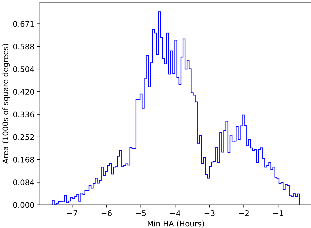
extra_ss_neo3_v3.4_10yrs All sky g band: Min HA
