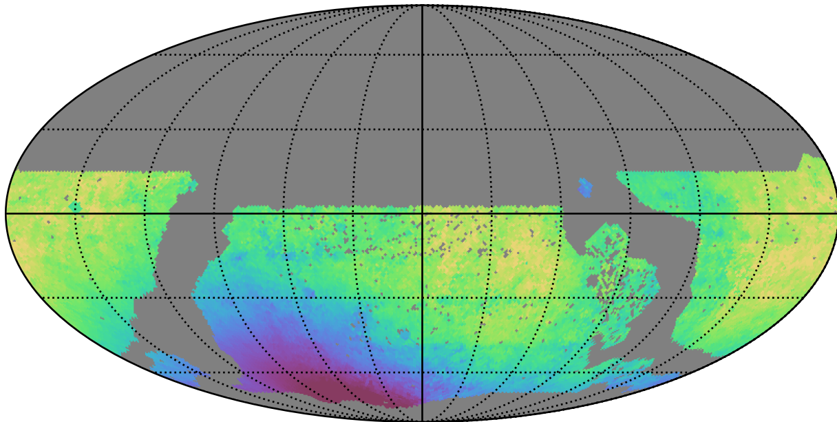
extra_ss_neo3_v3.4_10yrs WFD y band: Median solarElong
