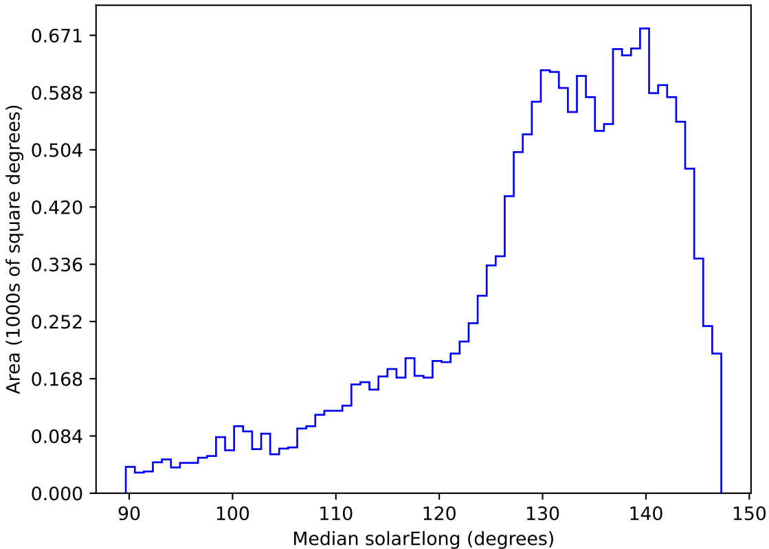
extra_ss_neo3_v3.4_10yrs WFD y band: Median solarElong
