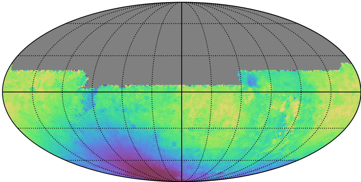
extra_ss_neo3_v3.4_10yrs All sky y band: Median solarElong
