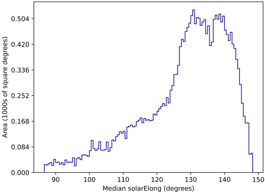
extra_ss_neo3_v3.4_10yrs All sky y band: Median solarElong
