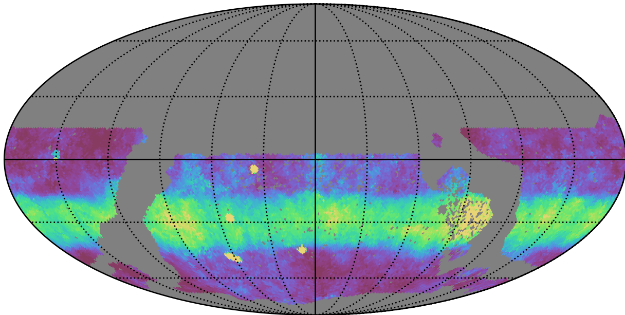
extra_ss_neo3_v3.4_10yrs WFD y band: Median normairmass
