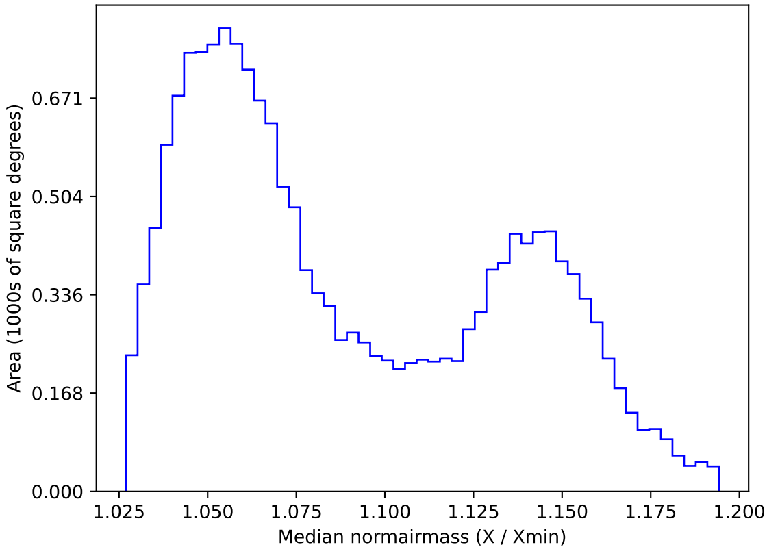
extra_ss_neo3_v3.4_10yrs WFD y band: Median normairmass
