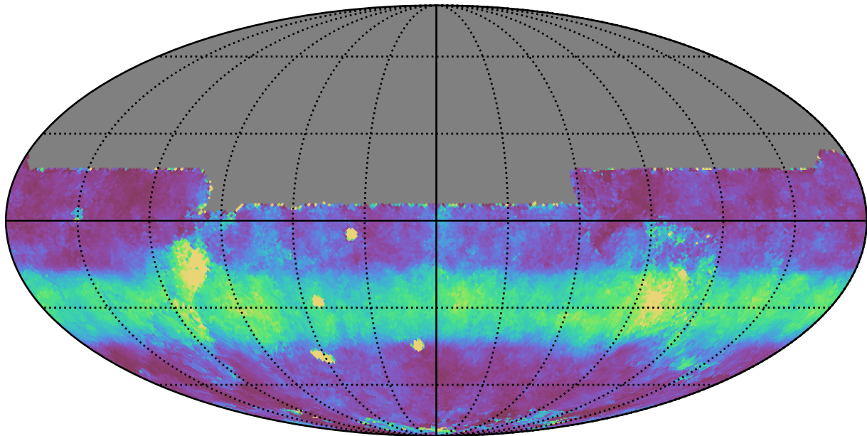
extra_ss_neo3_v3.4_10yrs All sky y band: Median normairmass
