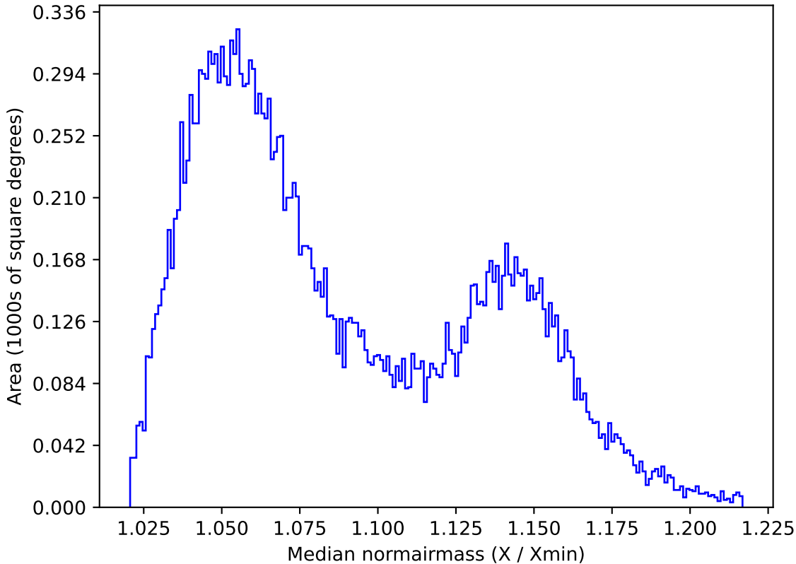
extra_ss_neo3_v3.4_10yrs All sky y band: Median normairmass
