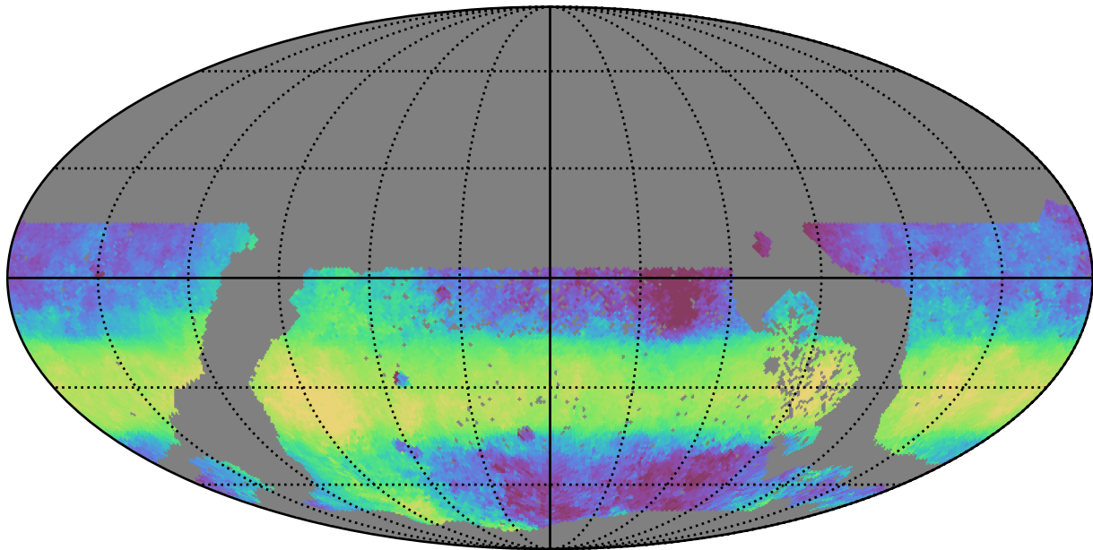
extra_ss_neo3_v3.4_10yrs WFD y band: Median HA
