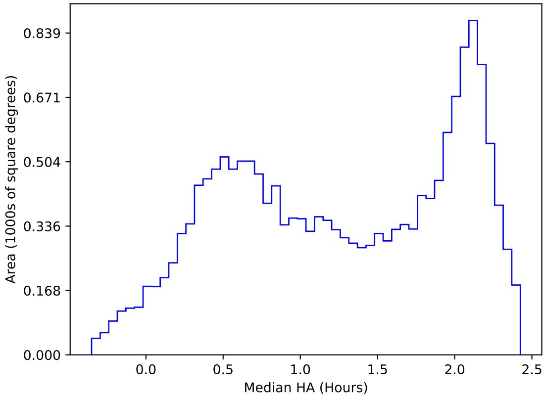
extra_ss_neo3_v3.4_10yrs WFD y band: Median HA
