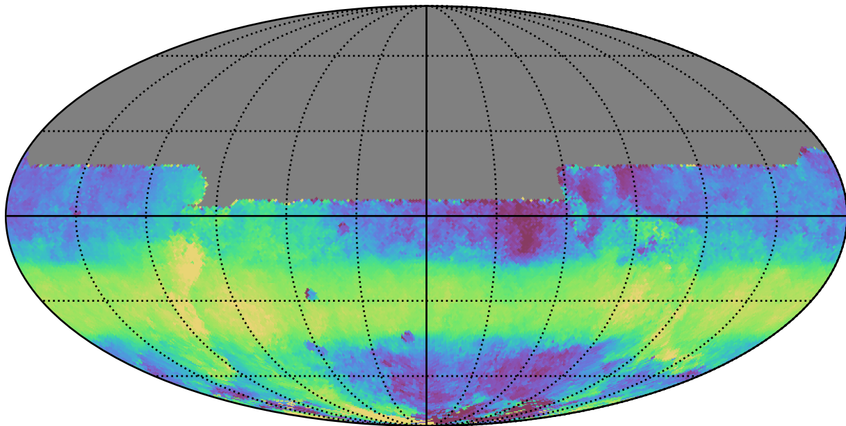
extra_ss_neo3_v3.4_10yrs All sky y band: Median HA
