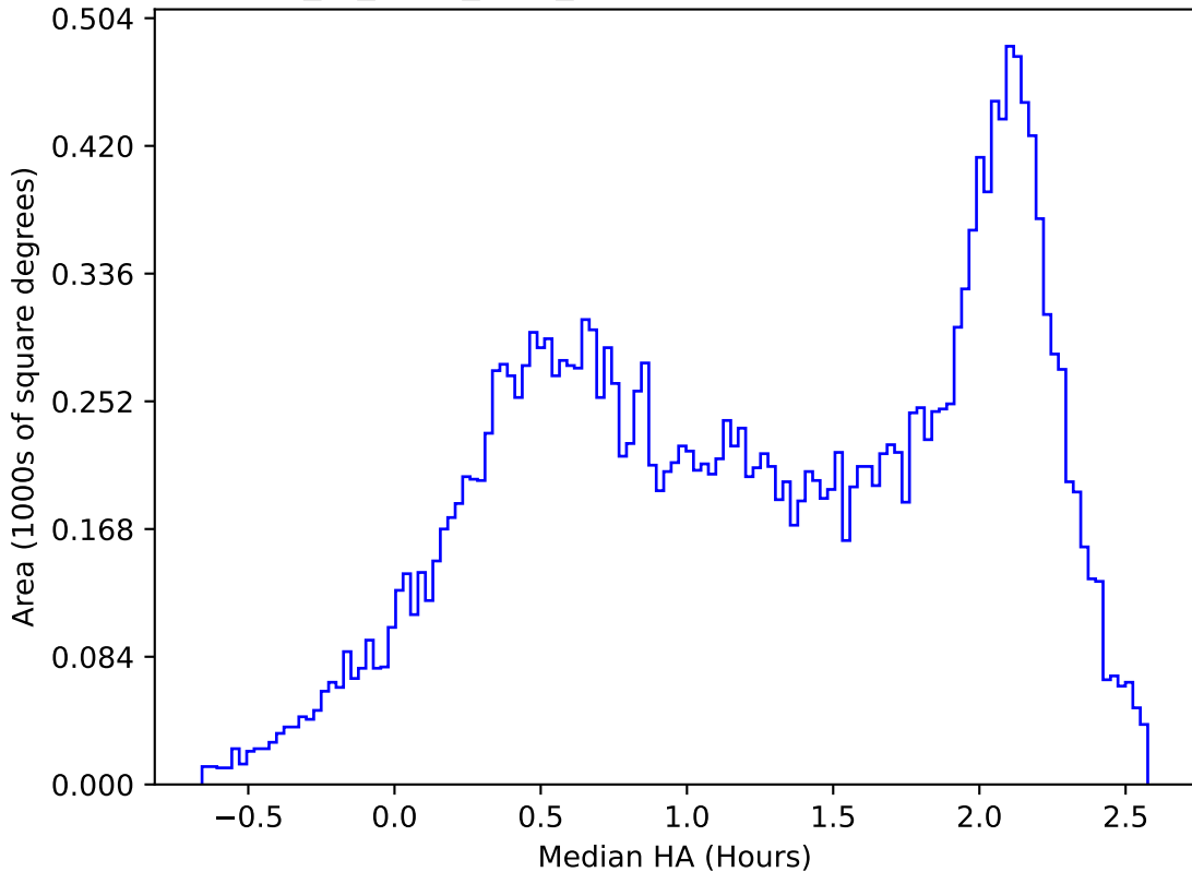
extra_ss_neo3_v3.4_10yrs All sky y band: Median HA
