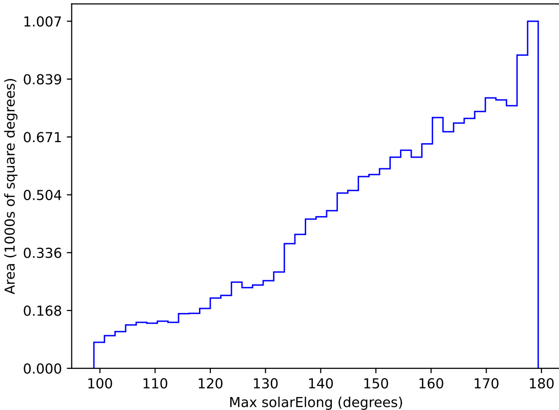
extra_ss_neo3_v3.4_10yrs WFD z band: Max solarElong
