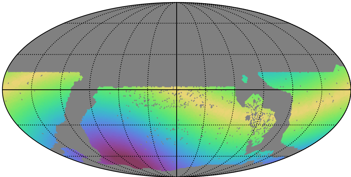
extra_ss_neo3_v3.4_10yrs WFD y band: Max solarElong
