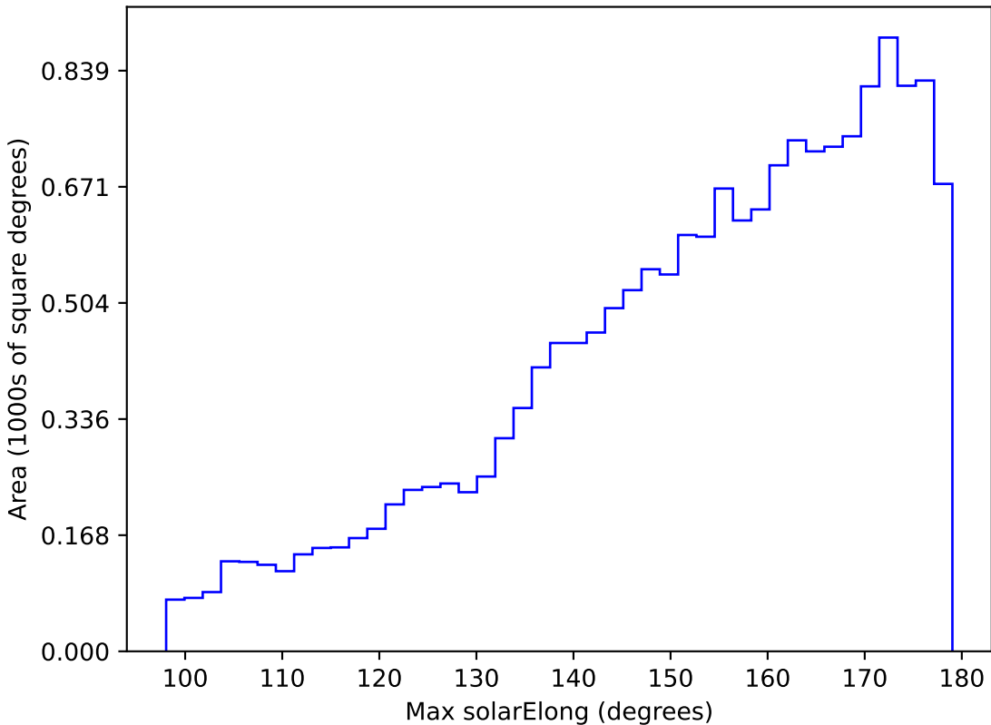
extra_ss_neo3_v3.4_10yrs WFD u band: Max solarElong
