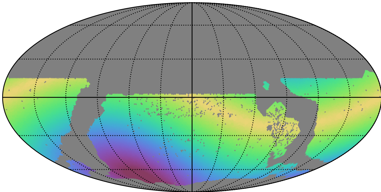
extra_ss_neo3_v3.4_10yrs WFD r band: Max solarElong
