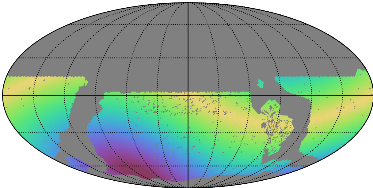
extra_ss_neo3_v3.4_10yrs WFD i band: Max solarElong
