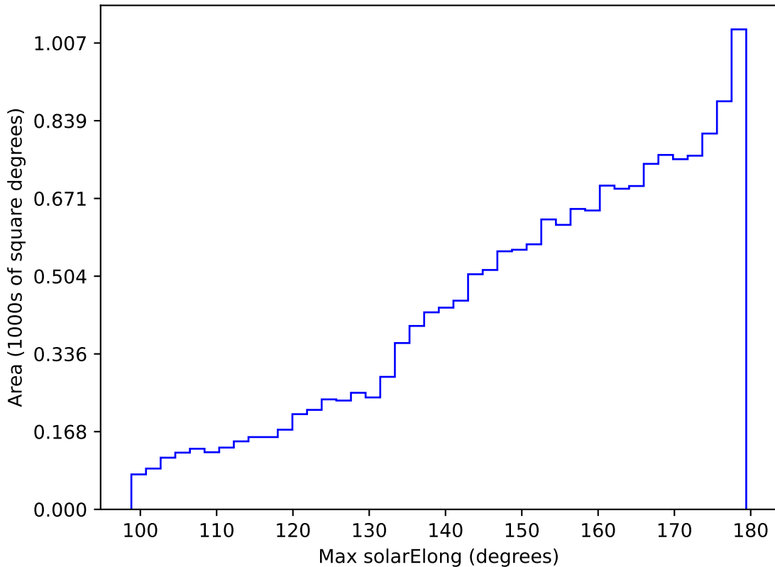
extra_ss_neo3_v3.4_10yrs WFD i band: Max solarElong
