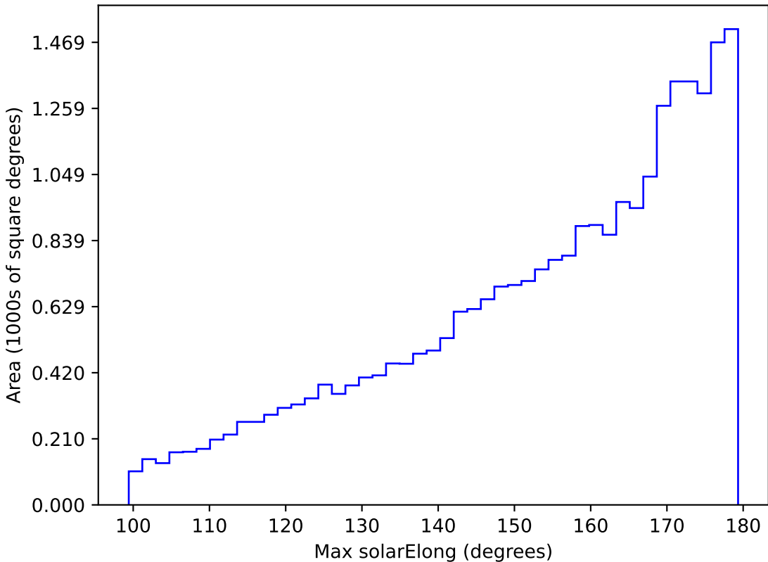
extra_ss_neo3_v3.4_10yrs All sky z band: Max solarElong
