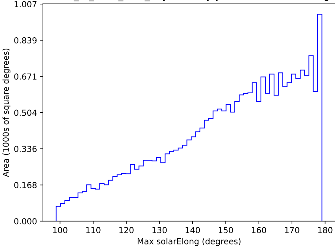
extra_ss_neo3_v3.4_10yrs All sky y band: Max solarElong
