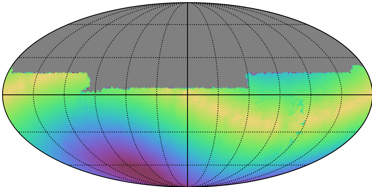
extra_ss_neo3_v3.4_10yrs All sky u band: Max solarElong
