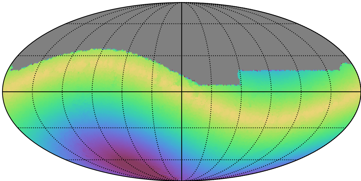
extra_ss_neo3_v3.4_10yrs All sky g band: Max solarElong
