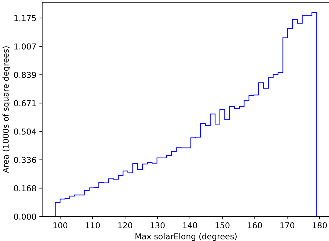
extra_ss_neo3_v3.4_10yrs All sky g band: Max solarElong
