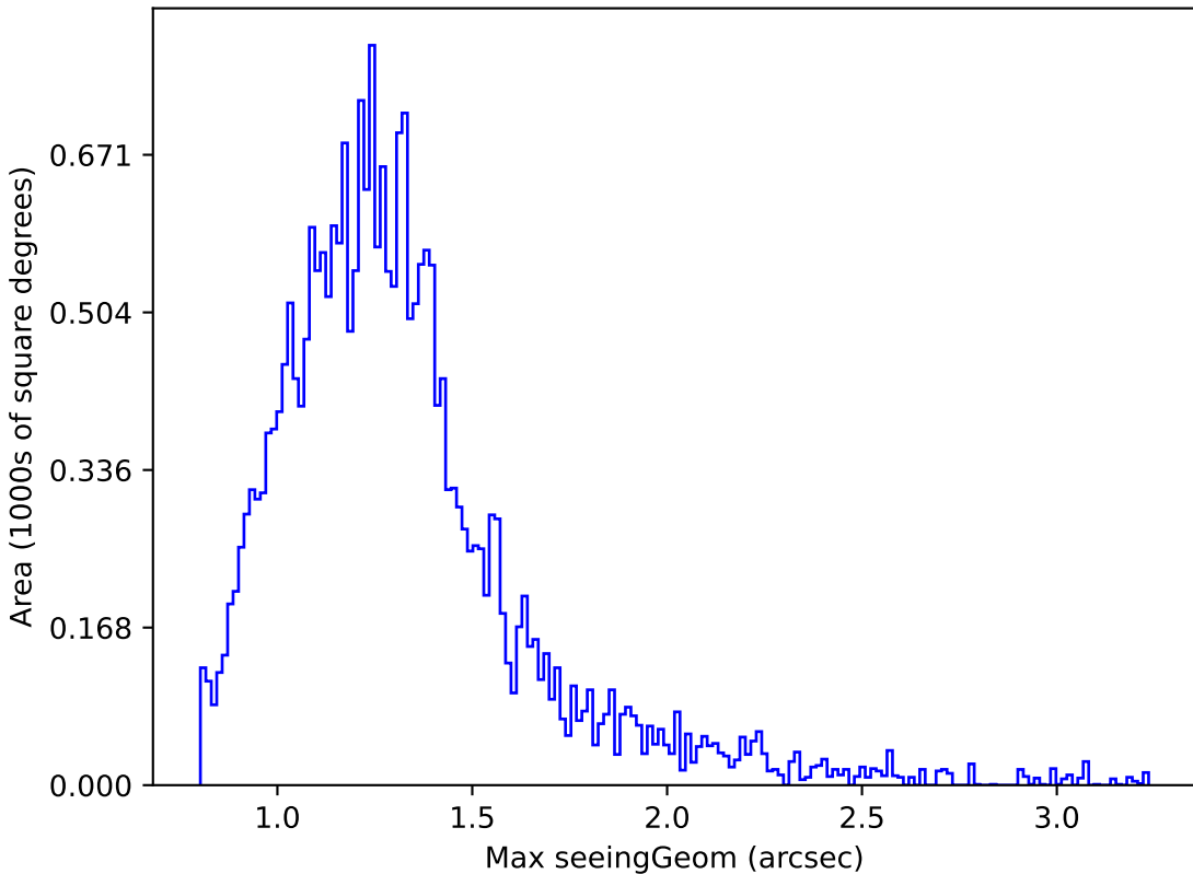
extra_ss_neo3_v3.4_10yrs Yr 1 z band: Max seeingGeom
