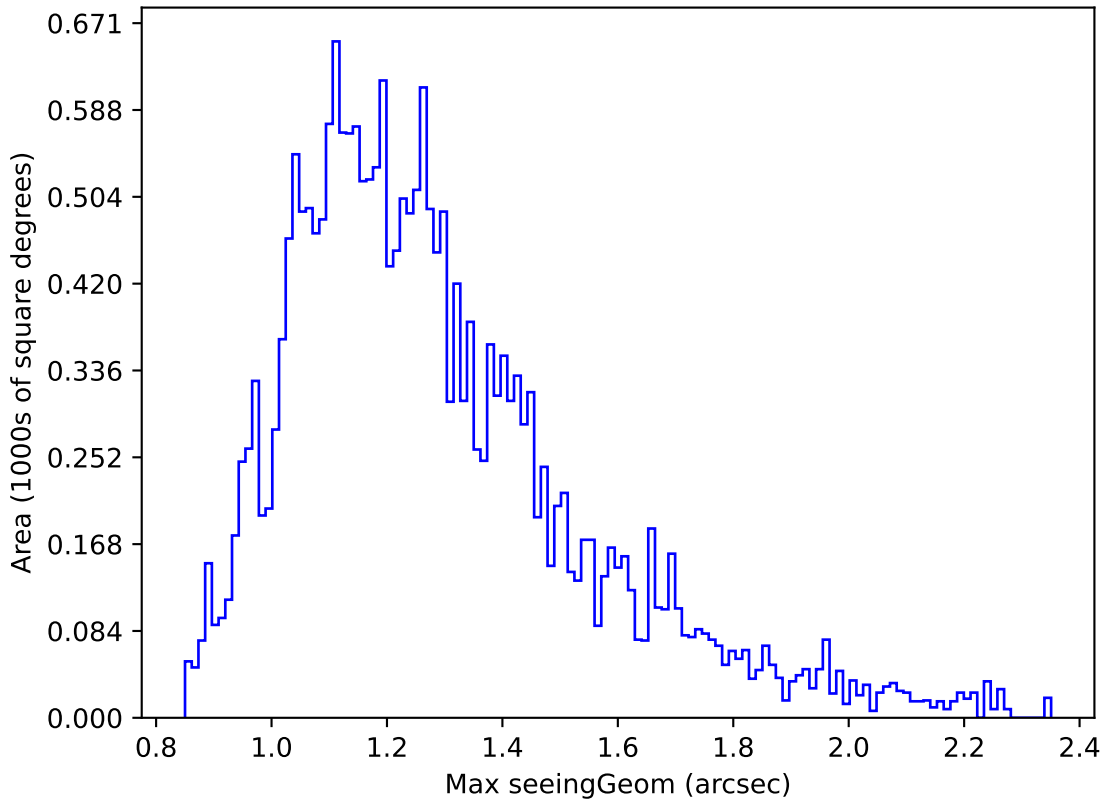
extra_ss_neo3_v3.4_10yrs Yr 1 y band: Max seeingGeom
