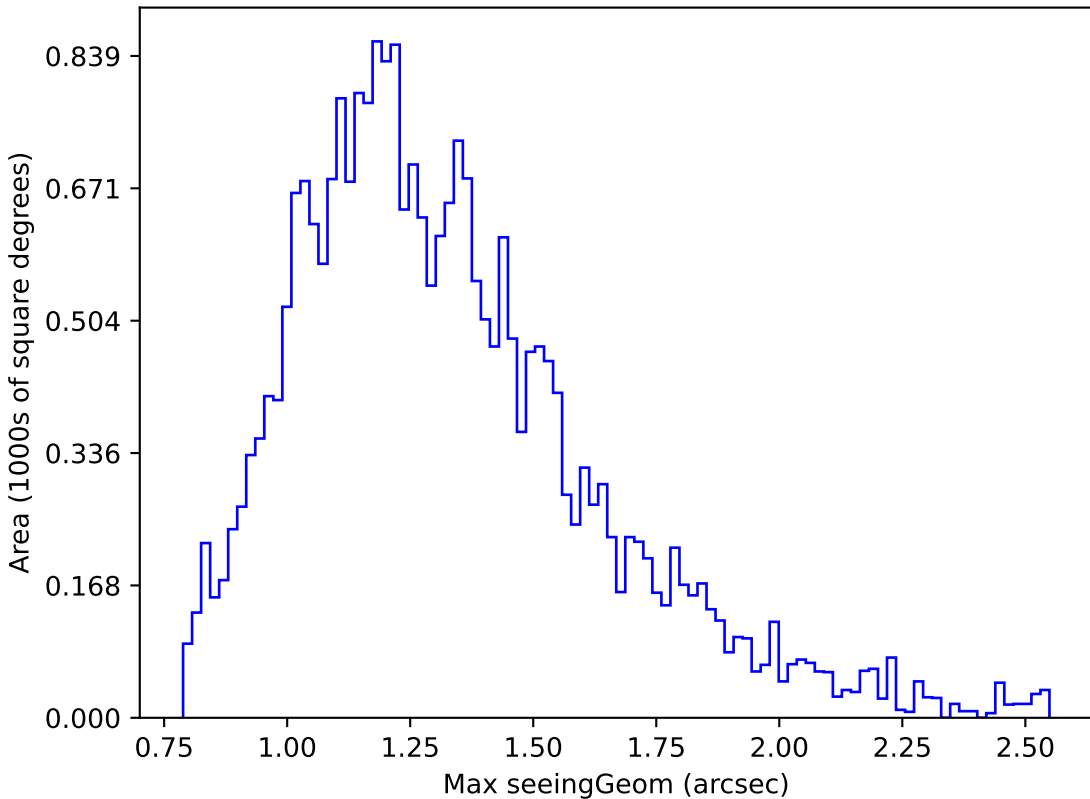
extra_ss_neo3_v3.4_10yrs Yr 1 i band: Max seeingGeom
