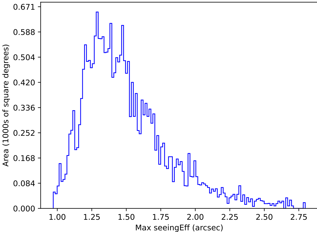
extra_ss_neo3_v3.4_10yrs Yr 1 y band: Max seeingEff
