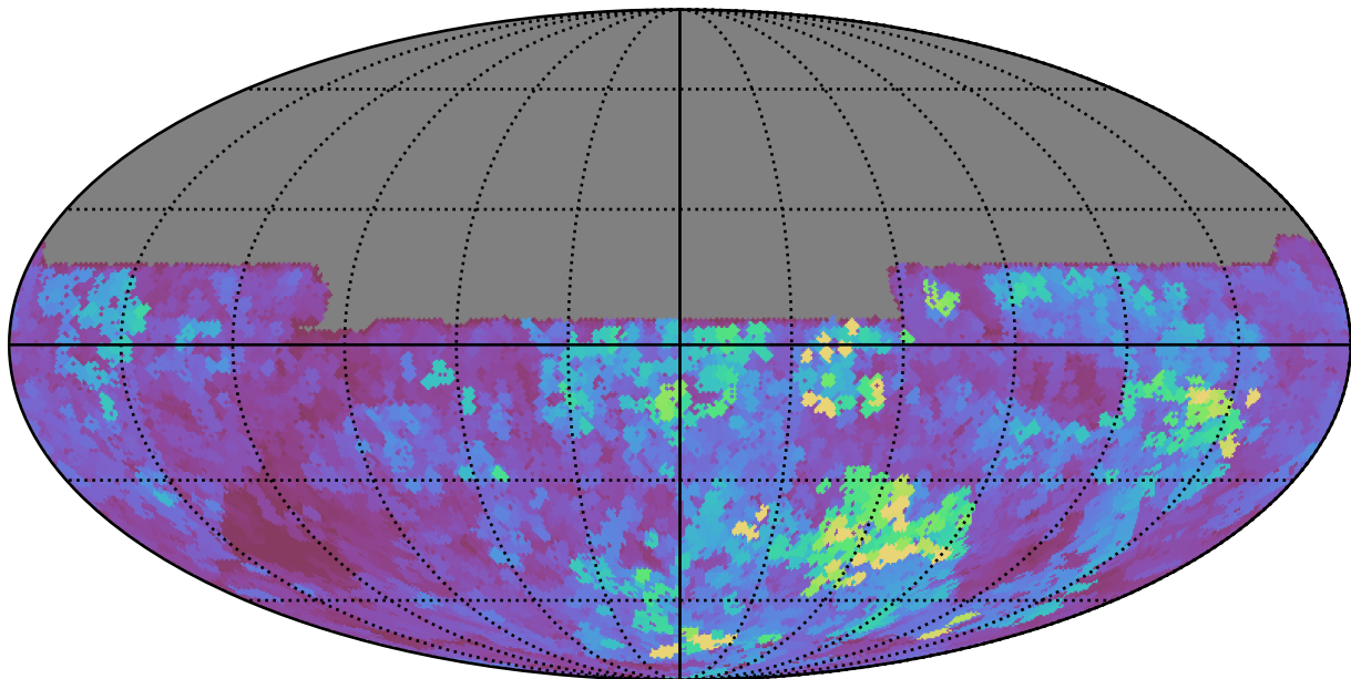
extra_ss_neo3_v3.4_10yrs All sky y band: Max seeingEff
