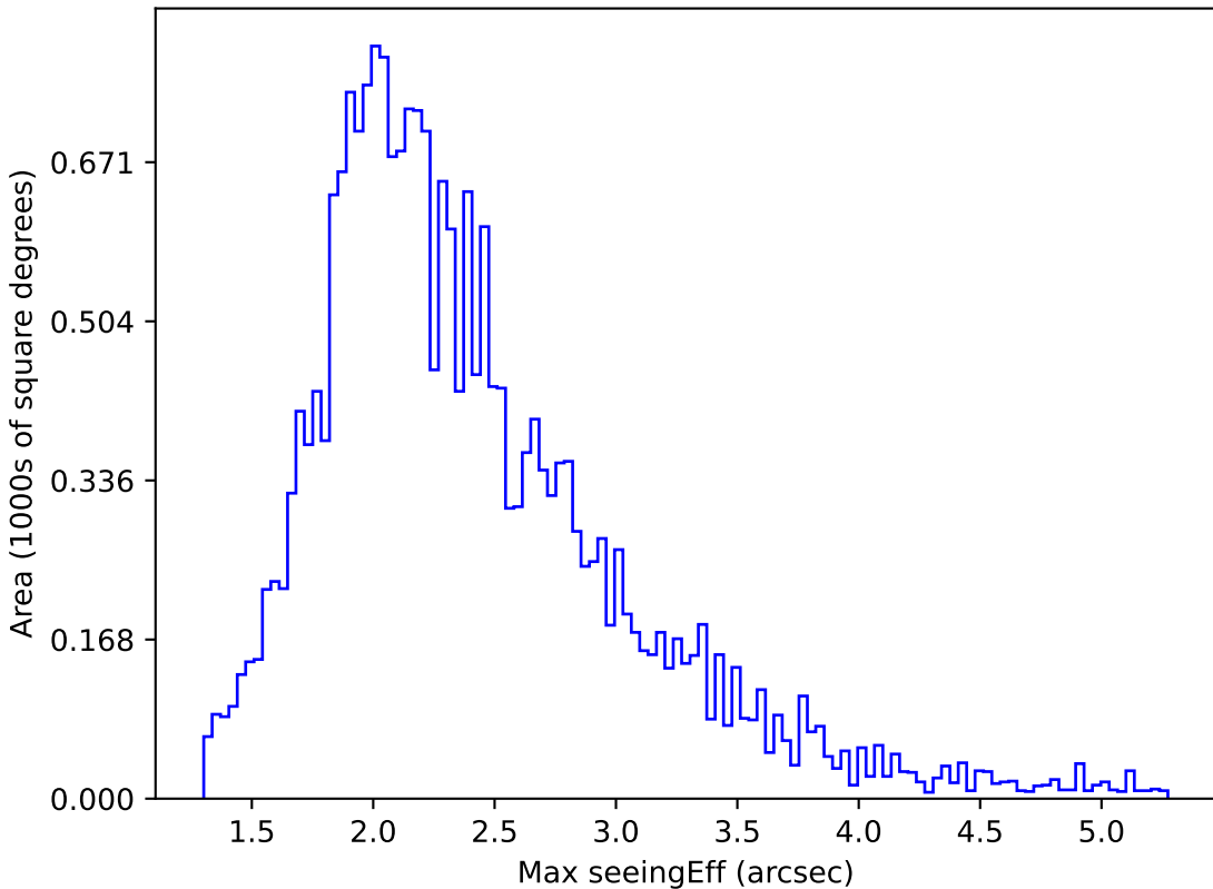
extra_ss_neo3_v3.4_10yrs All sky y band: Max seeingEff
