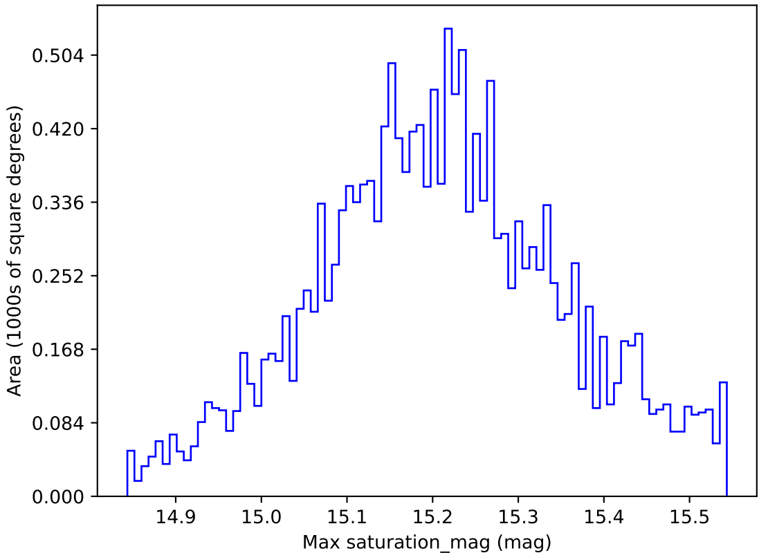
extra_ss_neo3_v3.4_10yrs WFD z band: Max saturation_mag
