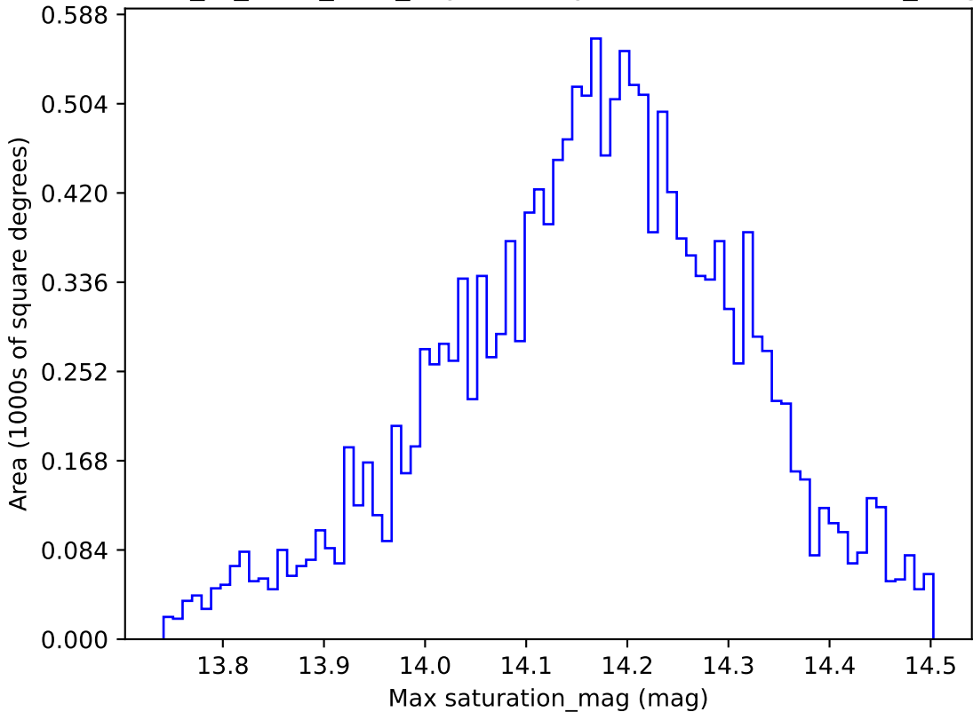
extra_ss_neo3_v3.4_10yrs WFD y band: Max saturation_mag
