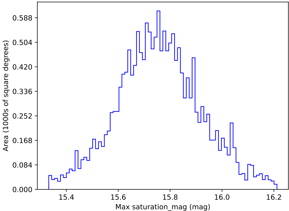
extra_ss_neo3_v3.4_10yrs WFD r band: Max saturation_mag
