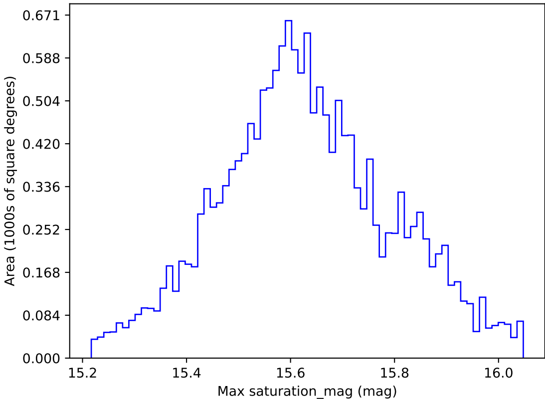
extra_ss_neo3_v3.4_10yrs WFD i band: Max saturation_mag
