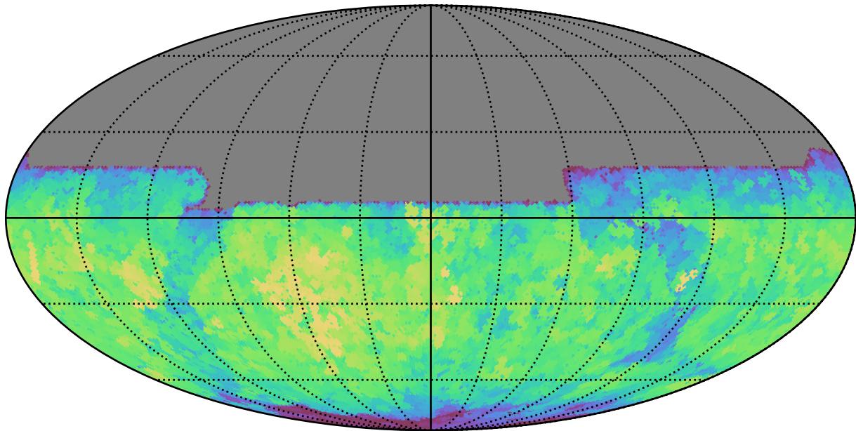
extra_ss_neo3_v3.4_10yrs All sky y band: Max saturation_mag
