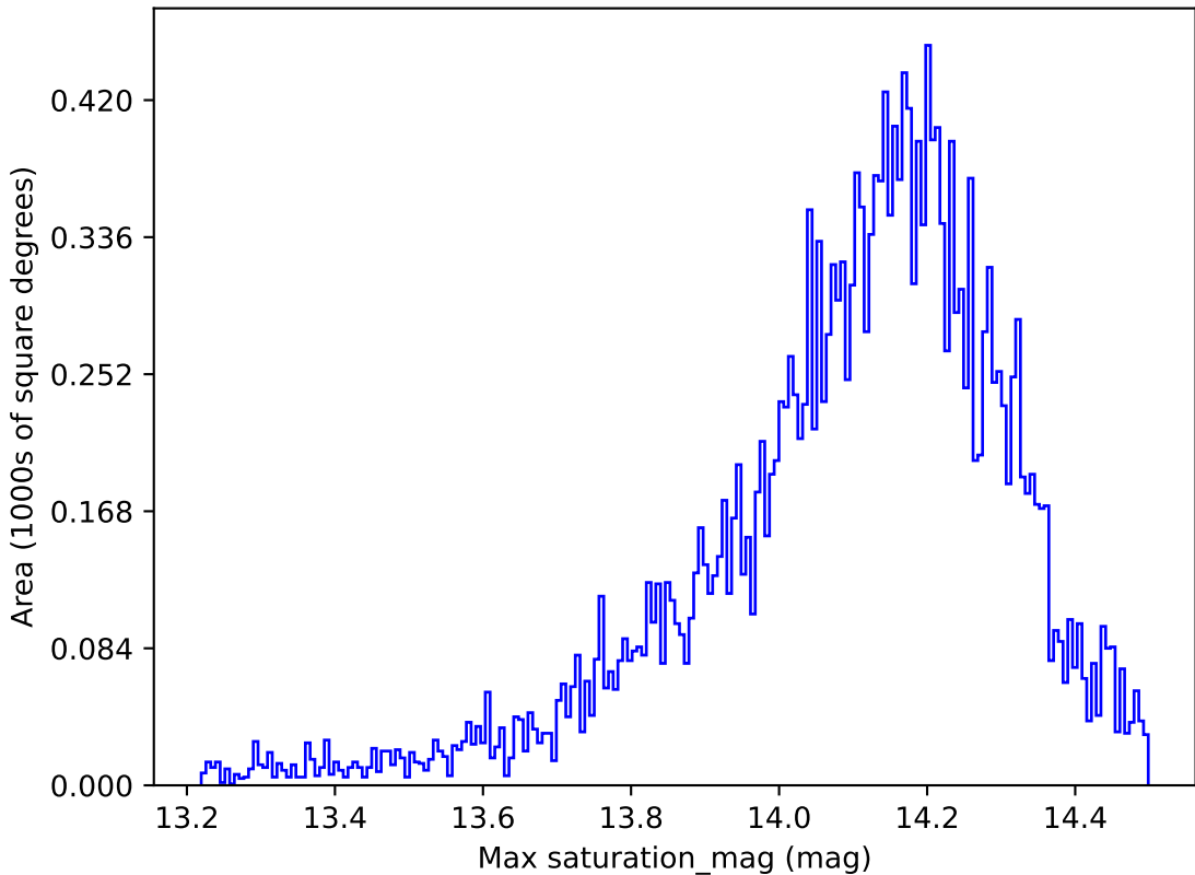
extra_ss_neo3_v3.4_10yrs All sky y band: Max saturation_mag
