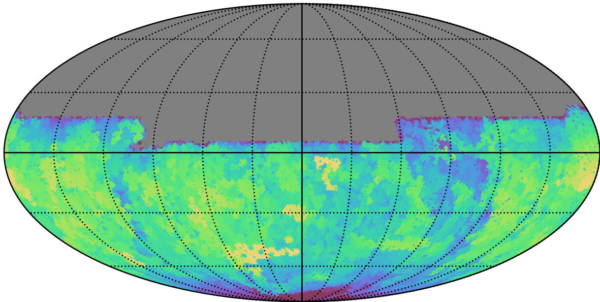
extra_ss_neo3_v3.4_10yrs All sky u band: Max saturation_mag
