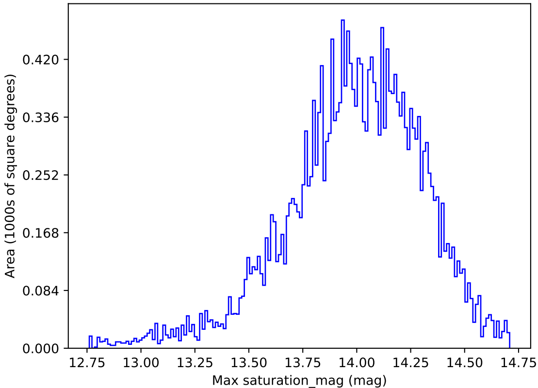
extra_ss_neo3_v3.4_10yrs All sky u band: Max saturation_mag
