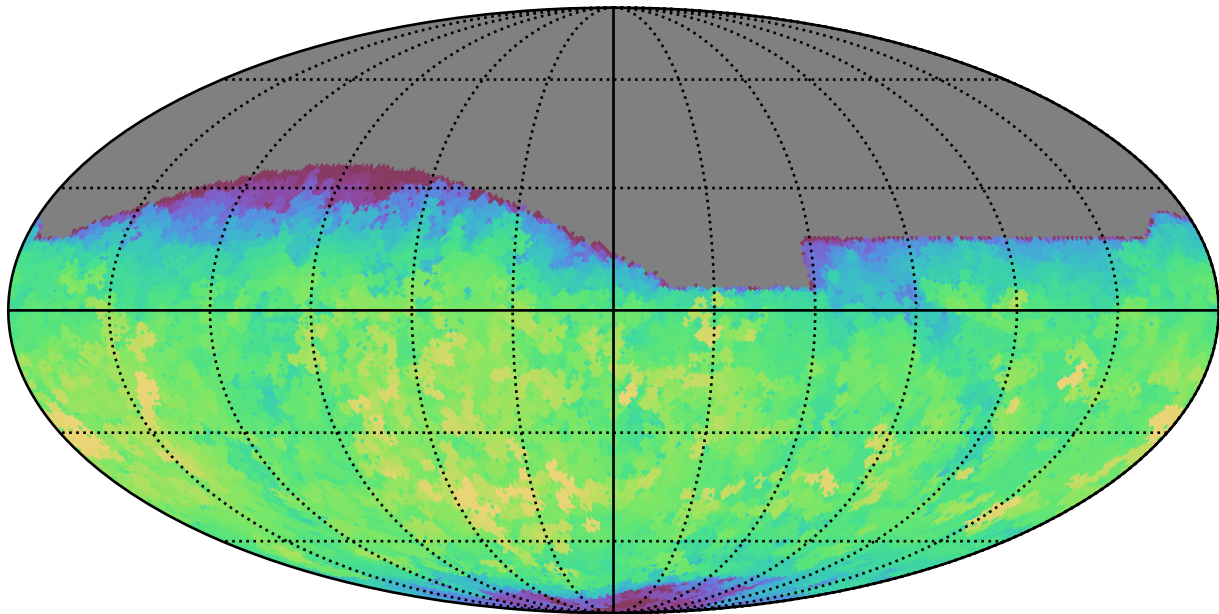
extra_ss_neo3_v3.4_10yrs All sky r band: Max saturation_mag
