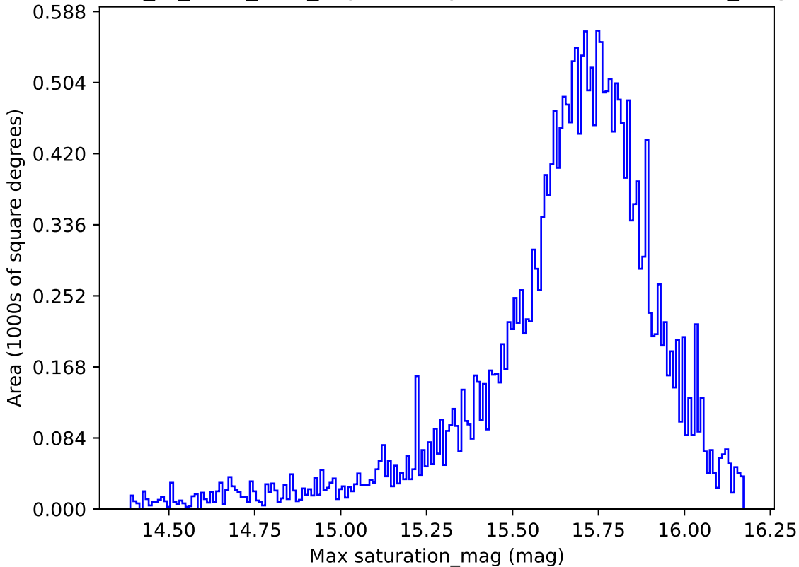
extra_ss_neo3_v3.4_10yrs All sky r band: Max saturation_mag
