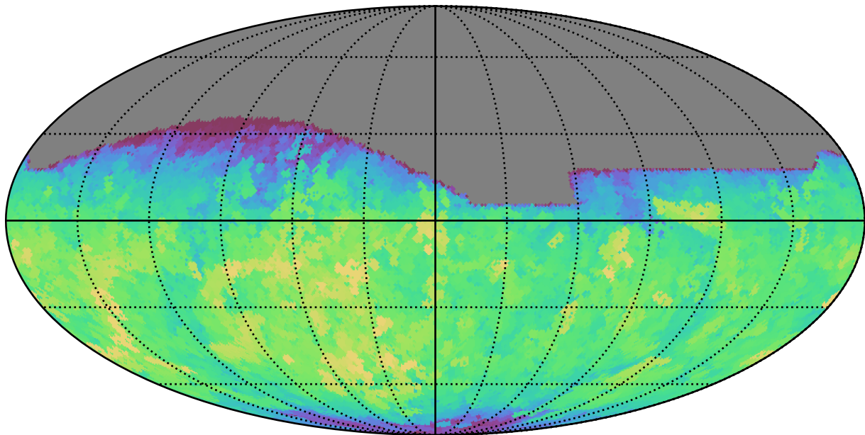
extra_ss_neo3_v3.4_10yrs All sky i band: Max saturation_mag
