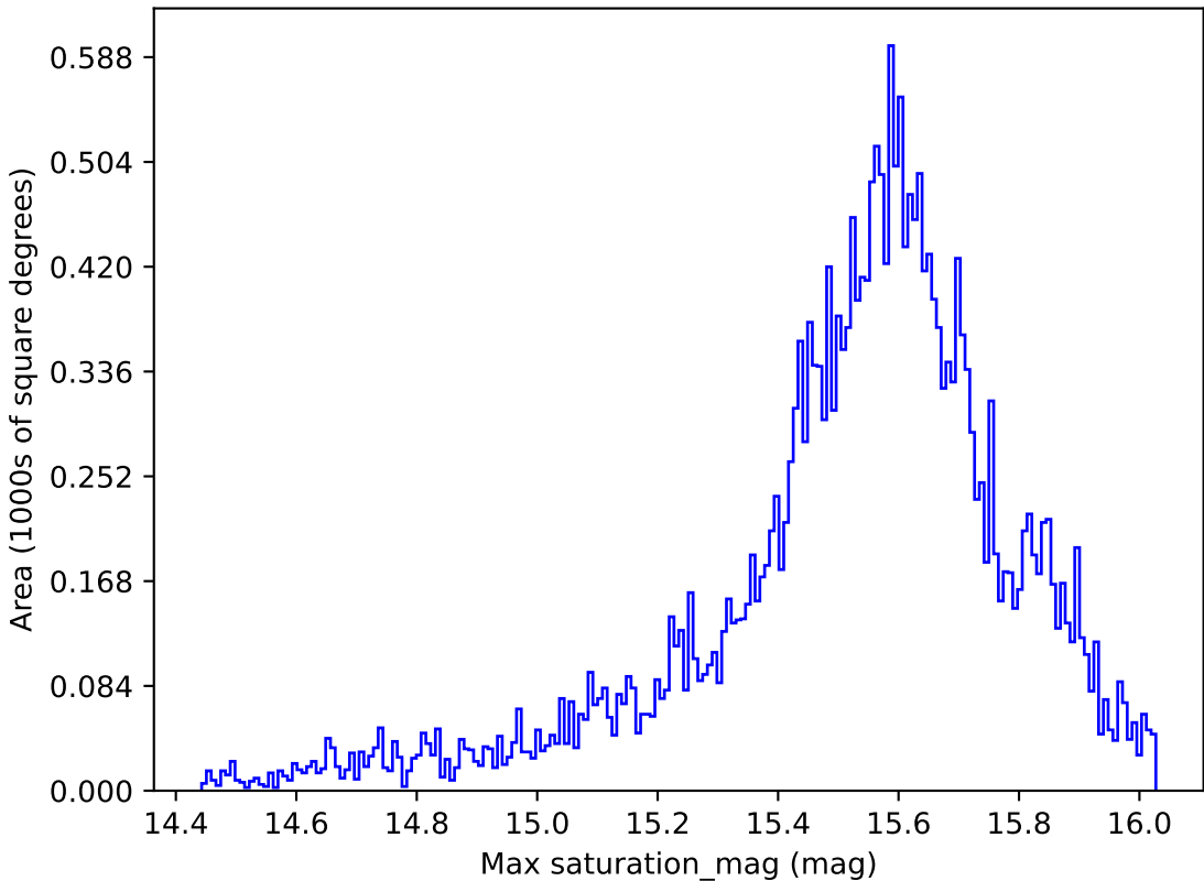
extra_ss_neo3_v3.4_10yrs All sky i band: Max saturation_mag
