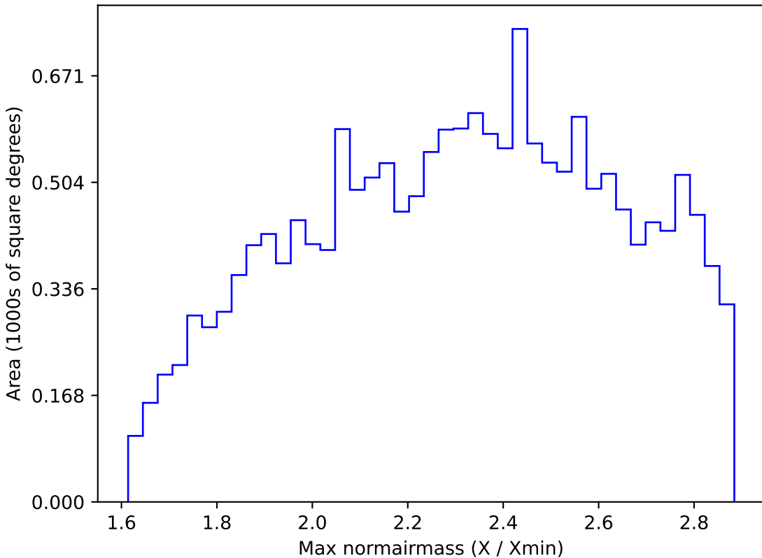
extra_ss_neo3_v3.4_10yrs WFD z band: Max normairmass
