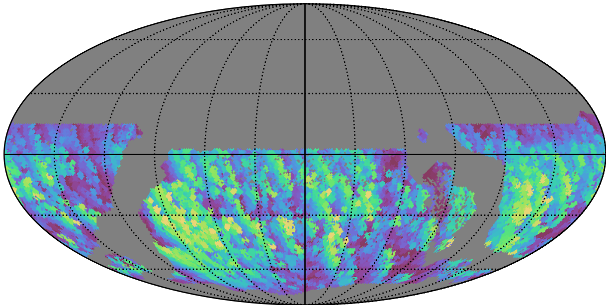
extra_ss_neo3_v3.4_10yrs WFD y band: Max normairmass
