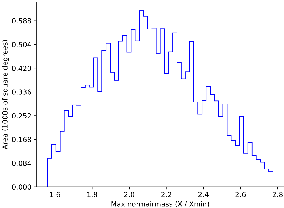
extra_ss_neo3_v3.4_10yrs WFD y band: Max normairmass
