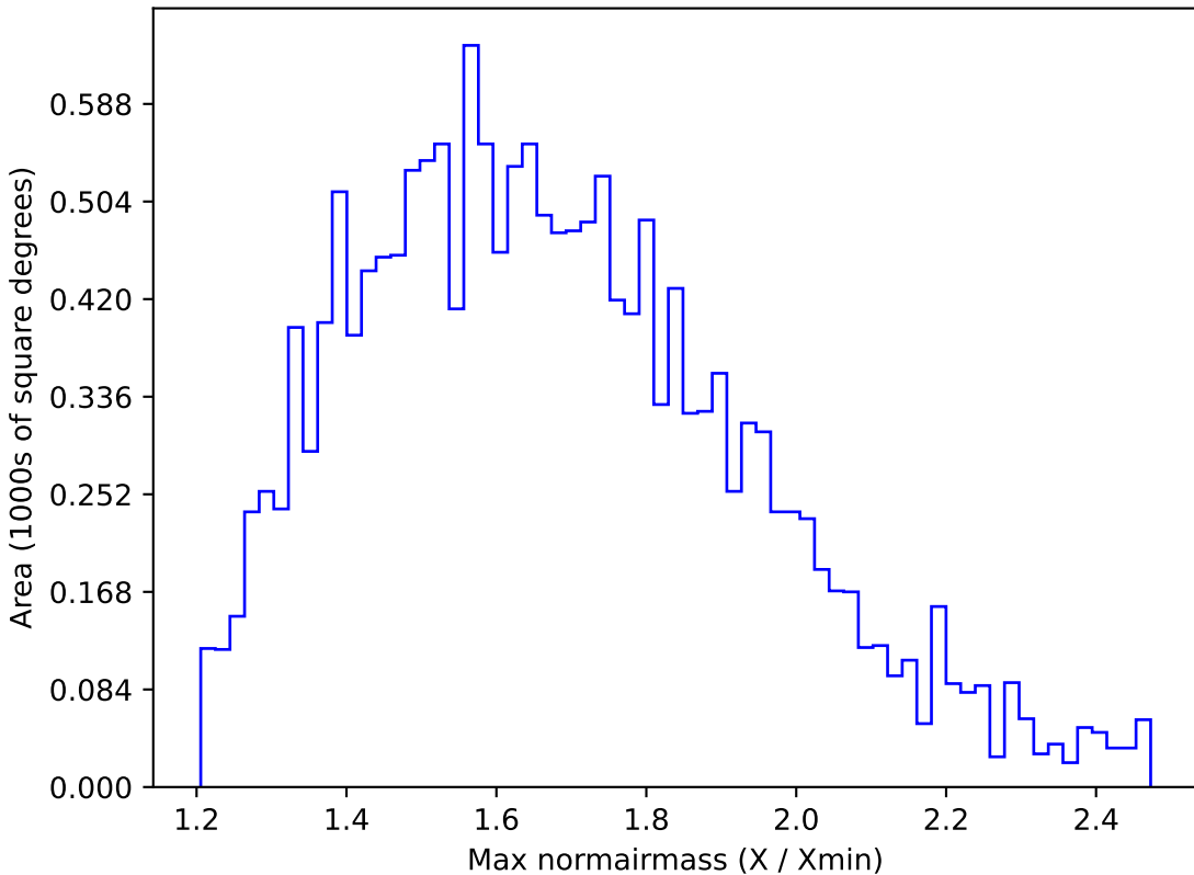
extra_ss_neo3_v3.4_10yrs WFD u band: Max normairmass
