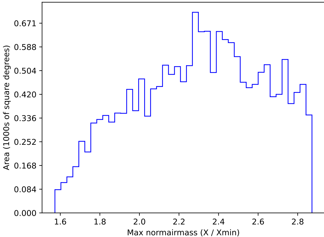
extra_ss_neo3_v3.4_10yrs WFD i band: Max normairmass
