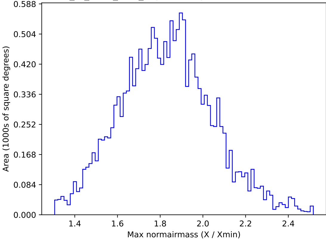
extra_ss_neo3_v3.4_10yrs WFD g band: Max normairmass
